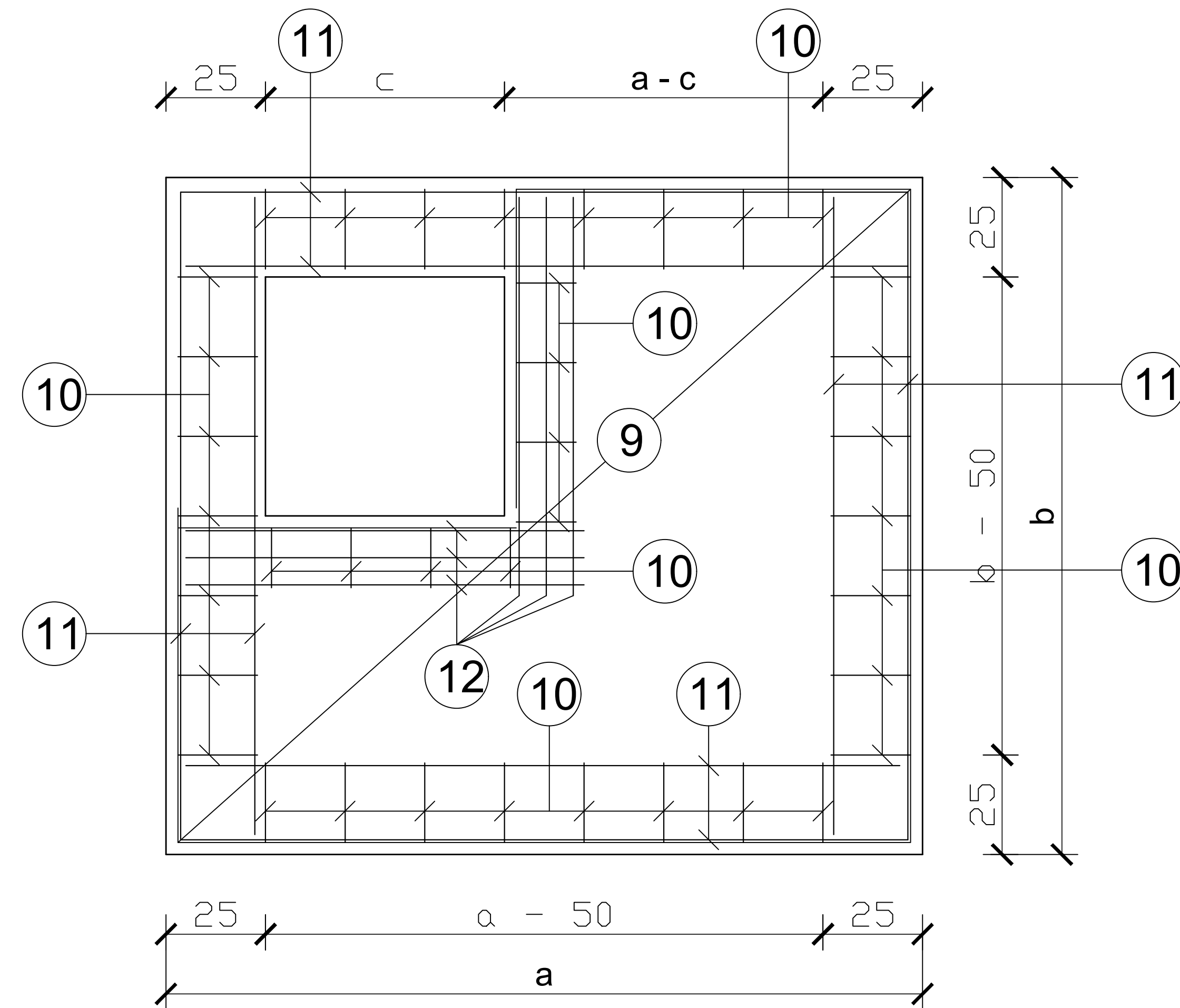
TLOCRT POKLOPNE PLOČE (PRESJEK C - C)
