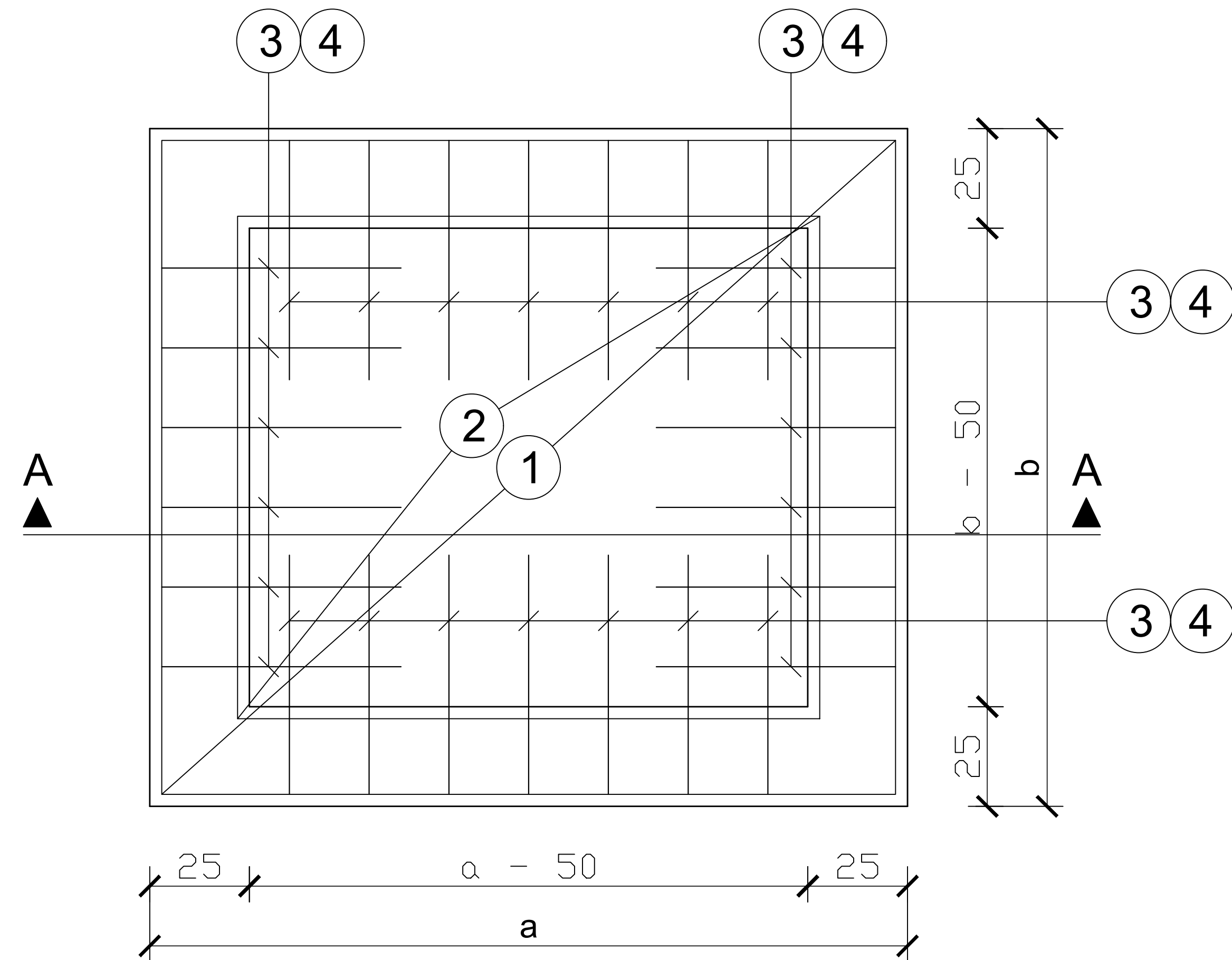
TLOCRT TEMELJNE PLOČE
